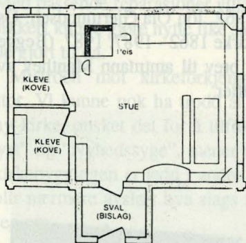
Akershusisk stue. Grunn- og møbleringsplan.
