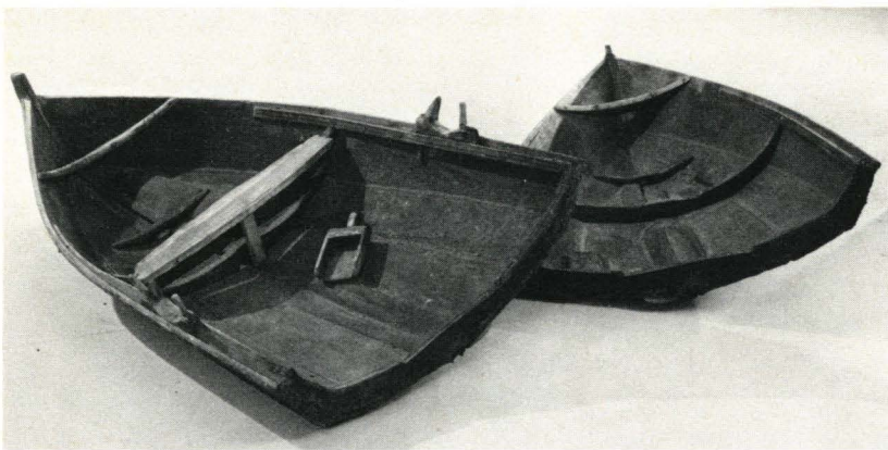
«Båt-Iva»-båten som kan deles i to og kløves til fjells.
