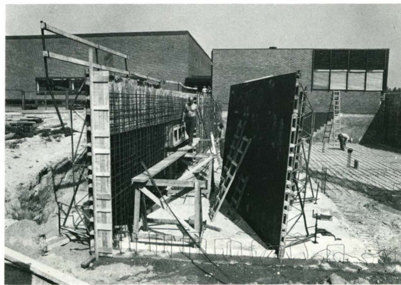
Forskaling og armering av veggene i tilbygget 2.8.78.
